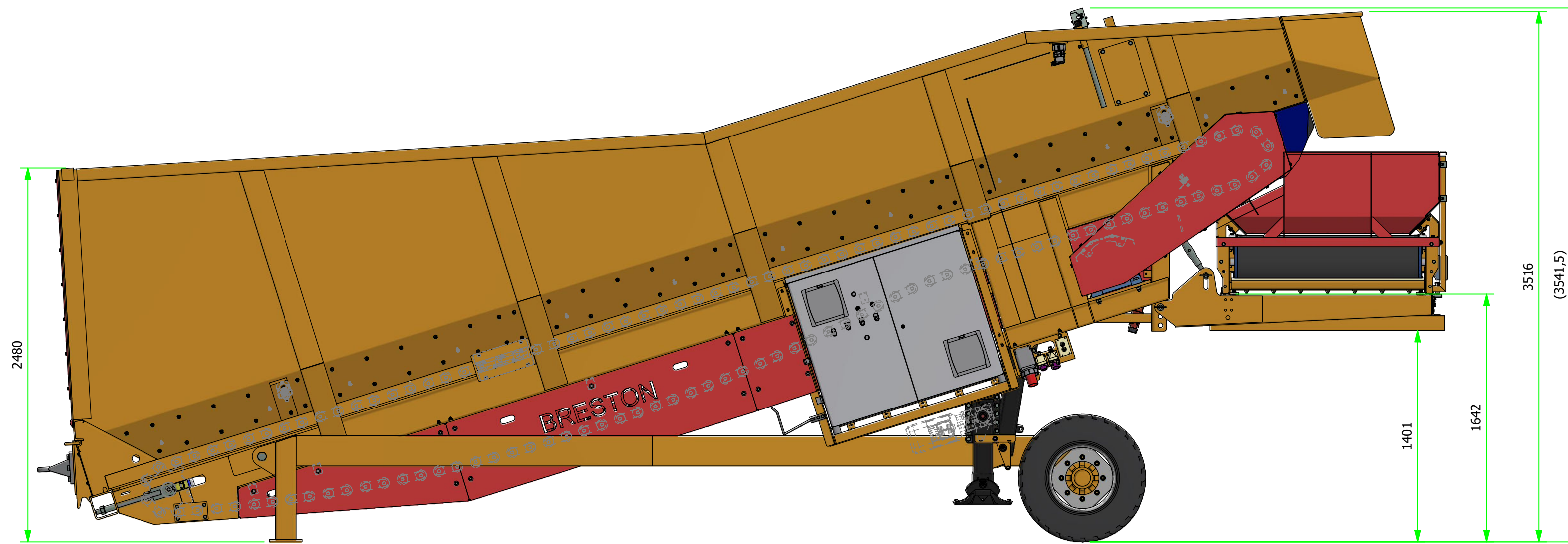
TRANSPORT STAND (1 : 25)
